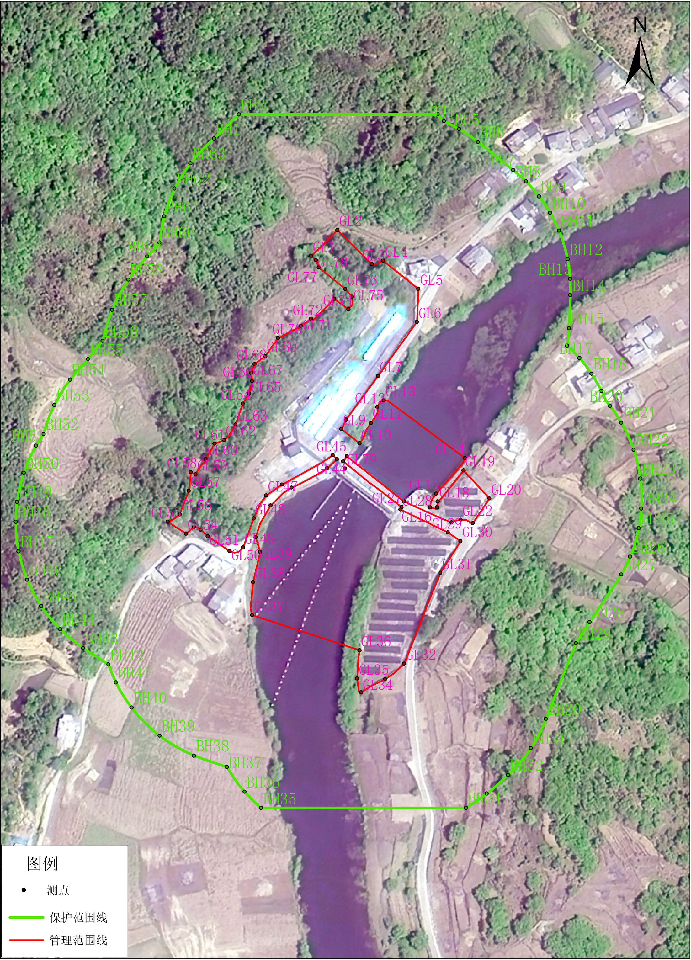
大寨水电站水库管理范围与保护范围划定平面图
